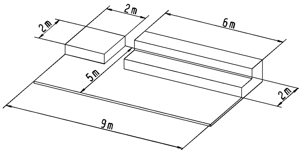
Zeichnung 1: Bühnengröße und -aufbau
